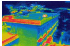
赤外線検査
